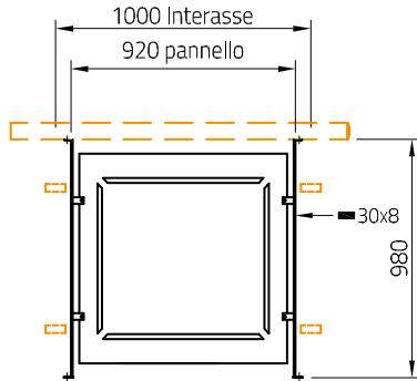
Terrazzo | Parapet LASER-T1010Z
