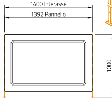
Recinzione | Fence LASER-R1410Z
